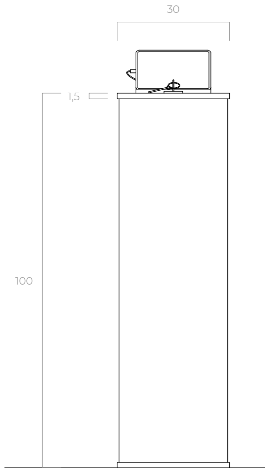
Prospetto frontale
