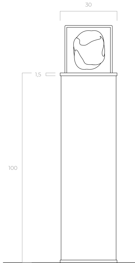
Prospetto frontale
